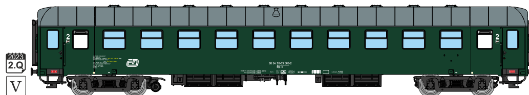
Osobní vůz Bp-k ČD Ústí nad Labem Personenwagen Bp-k ČD Ústí nad Labem
